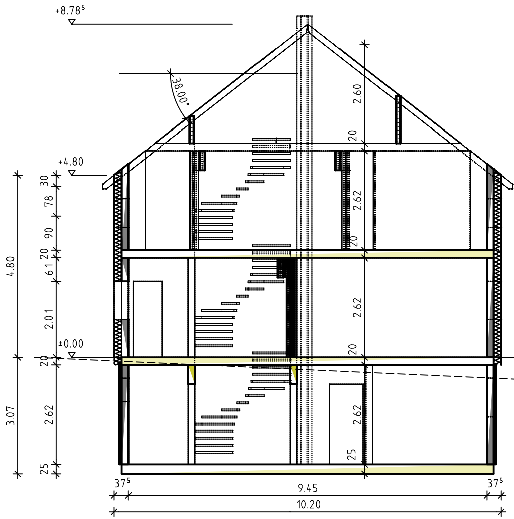
Vertikalschnitt M= 1: 100
